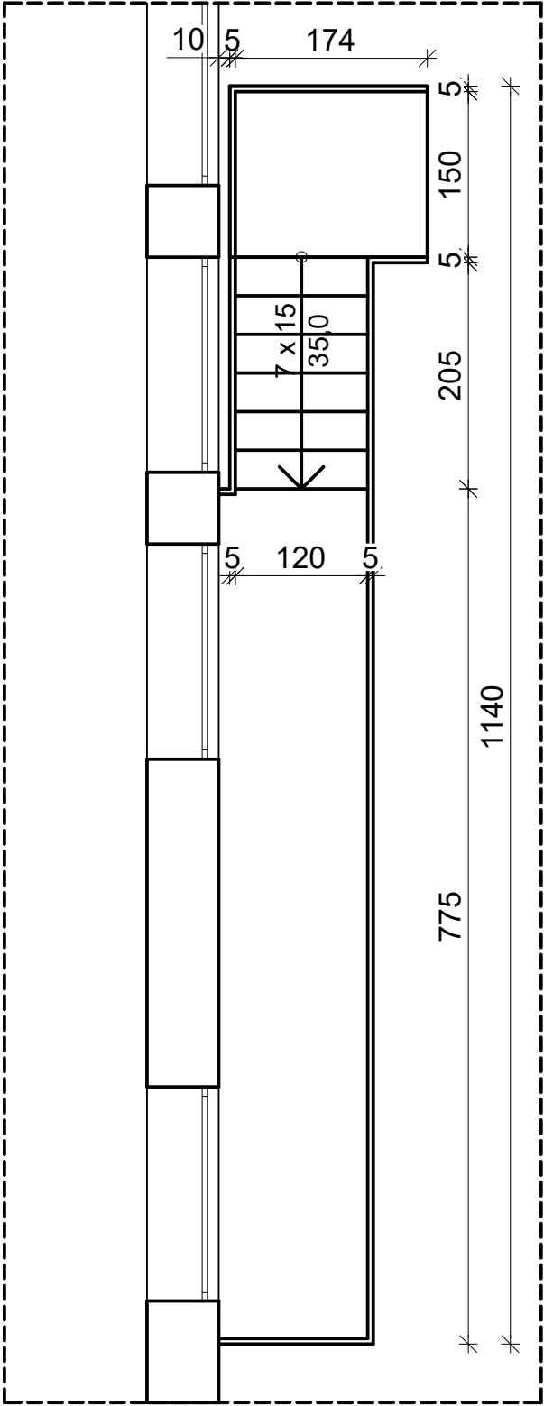
Rzut platformy
