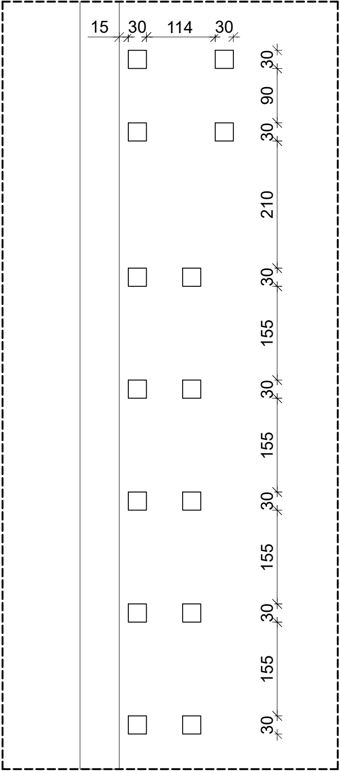
Rzut fundamentów platformy
